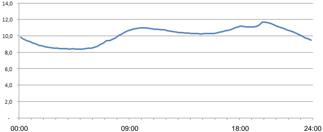
Elektrisch vermogen Nederland (GW)
